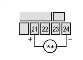
Figura 6 - conexão de tensão 5Vdc
