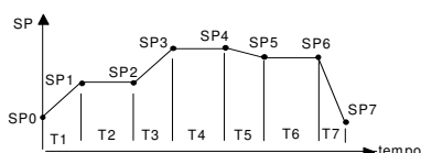
Figura 8 - Exemplo de programa de rampas e patamares
