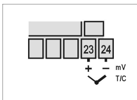
Figura 3 - conexão de Termopar e 0-50mV
