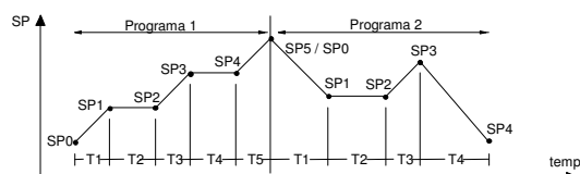
Figura 10 - Exemplo de programa 1 e 2 "linkados" (interligados)
